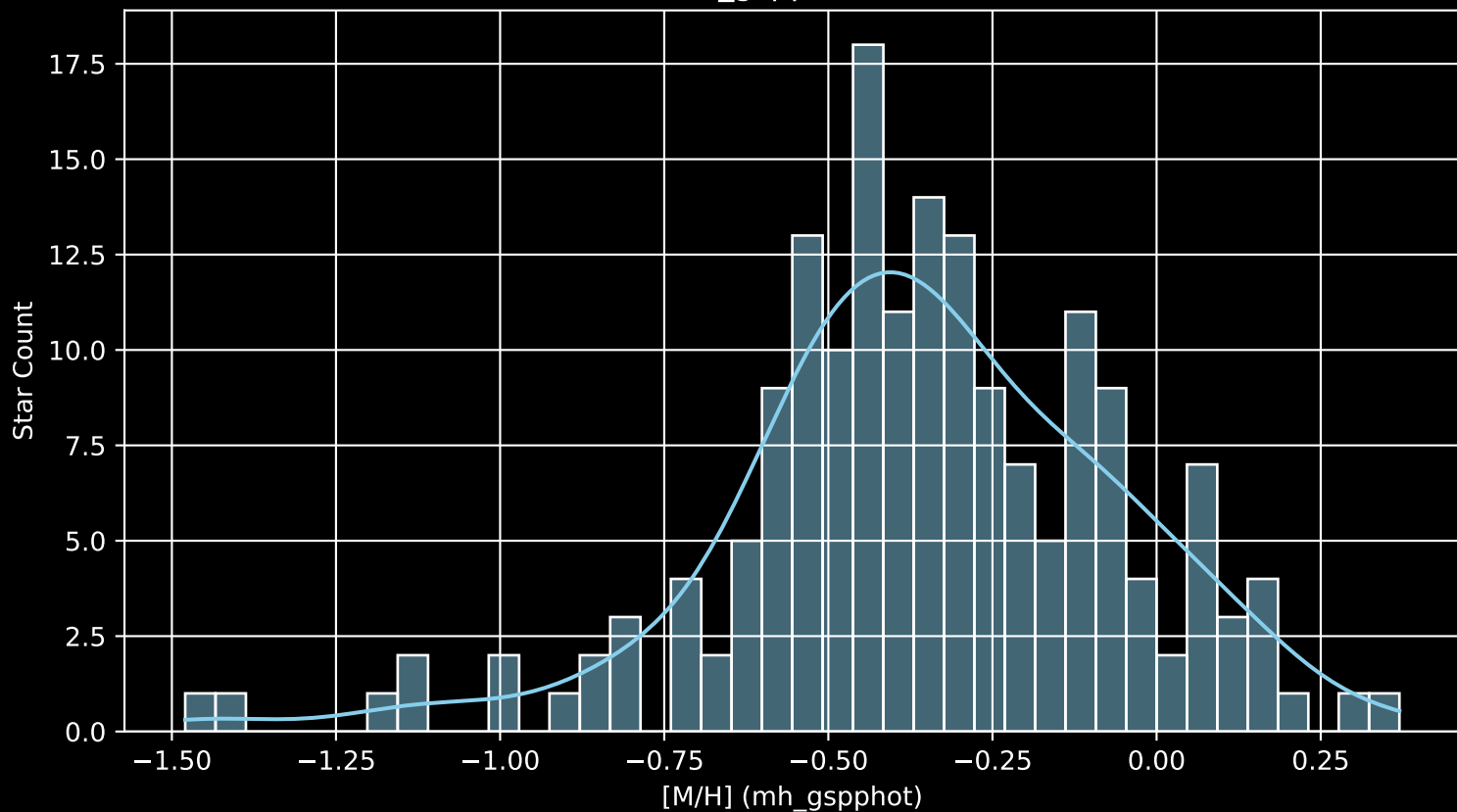
GALAH DR4 Field: [208] [M/H] (mh_gspphot) (n= 176)
