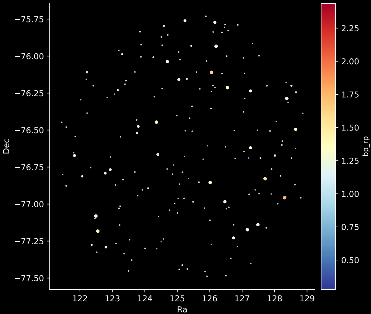
GALAH DR4 Field: [208] Stars: 176
