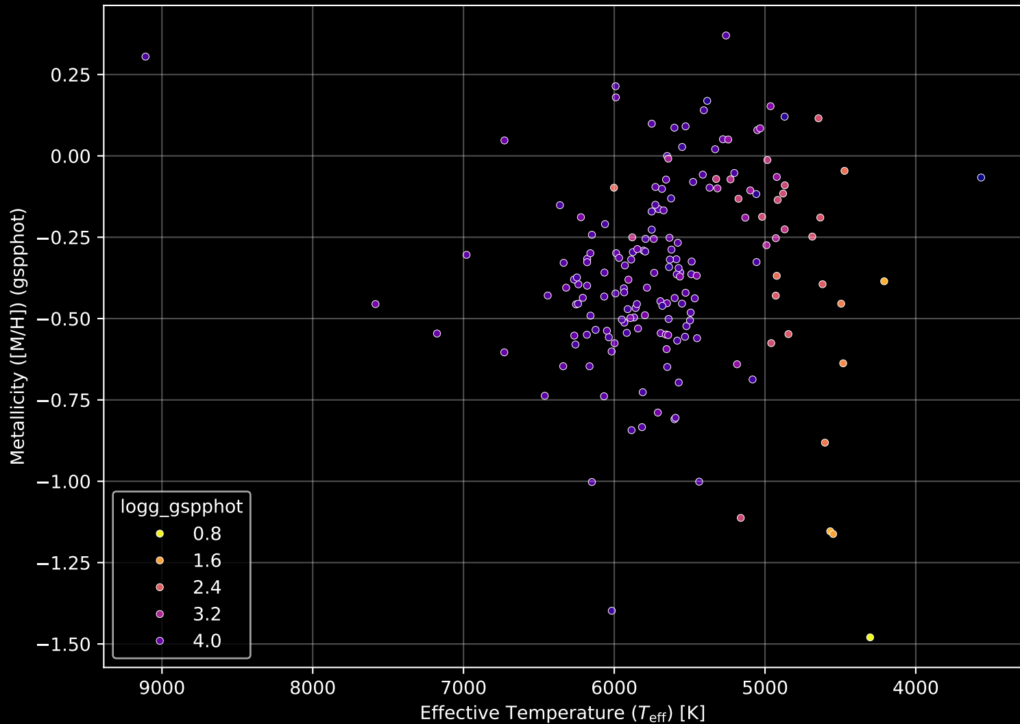
GALAH DR4 Field: [208] Stellar Population Parameters (n= 176)
