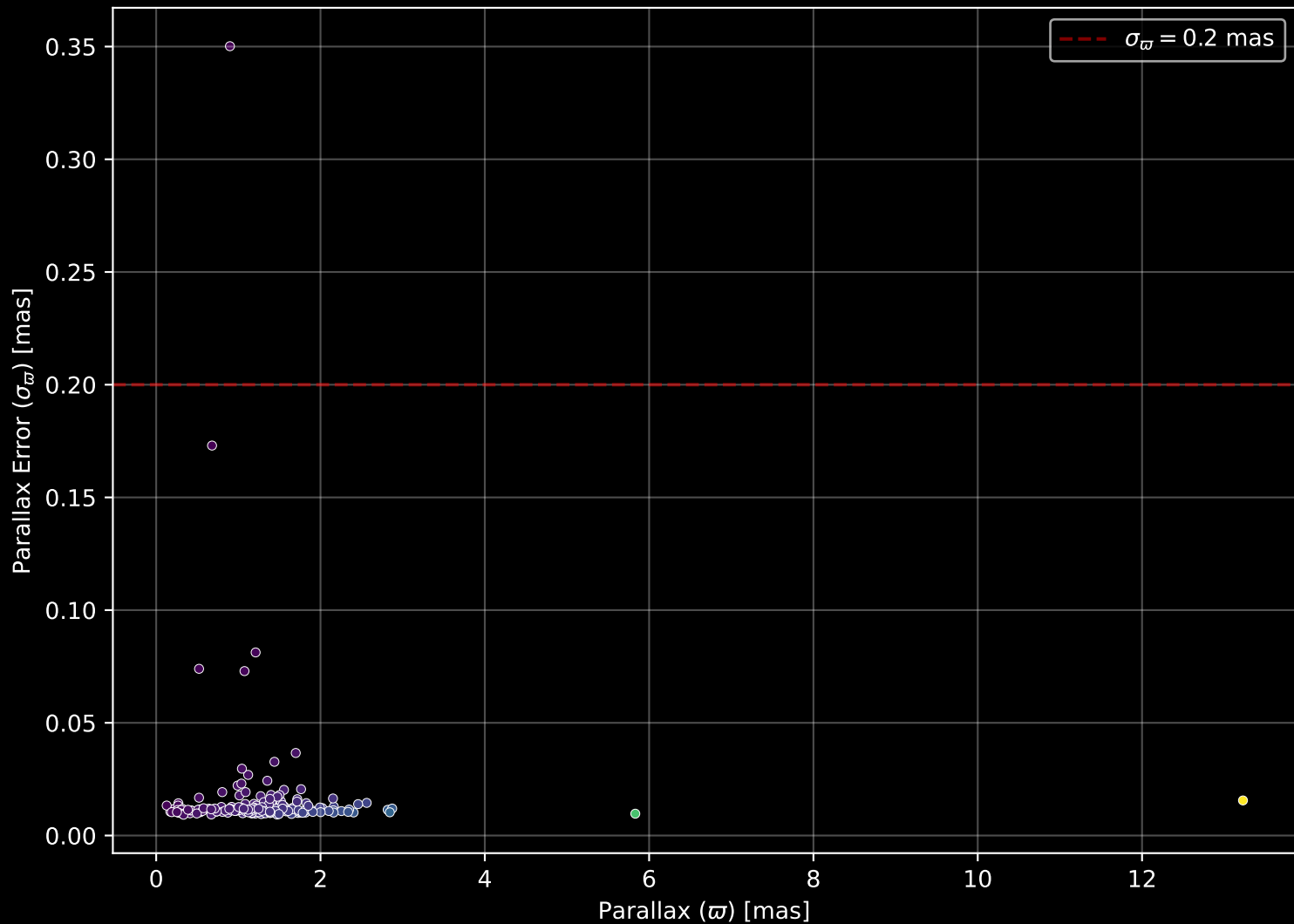
GALAH DR4 Field: [208] Parallax Quality (n= 176)
