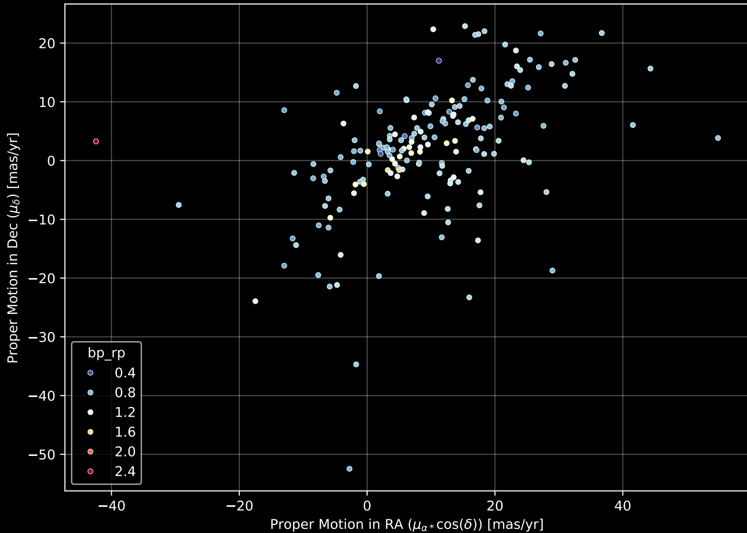
GALAH DR4 Field: [208] Proper Motion Diagram (n= 176)
